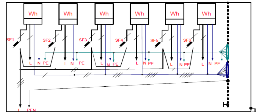
Įvadinės apskaitos spintos skirtos šešiems vienfaziams elektros skaitikliams įrengti principinė elektros schema
